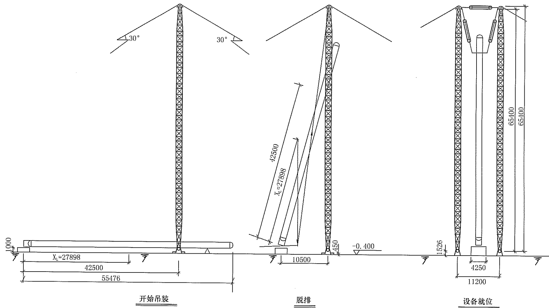
图 20.3.4 双桅杆吊装示意
