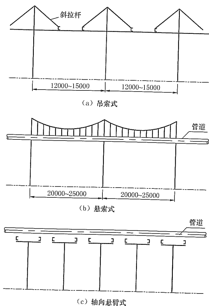
图 12.3.3 管架的连系结构型式(二)
