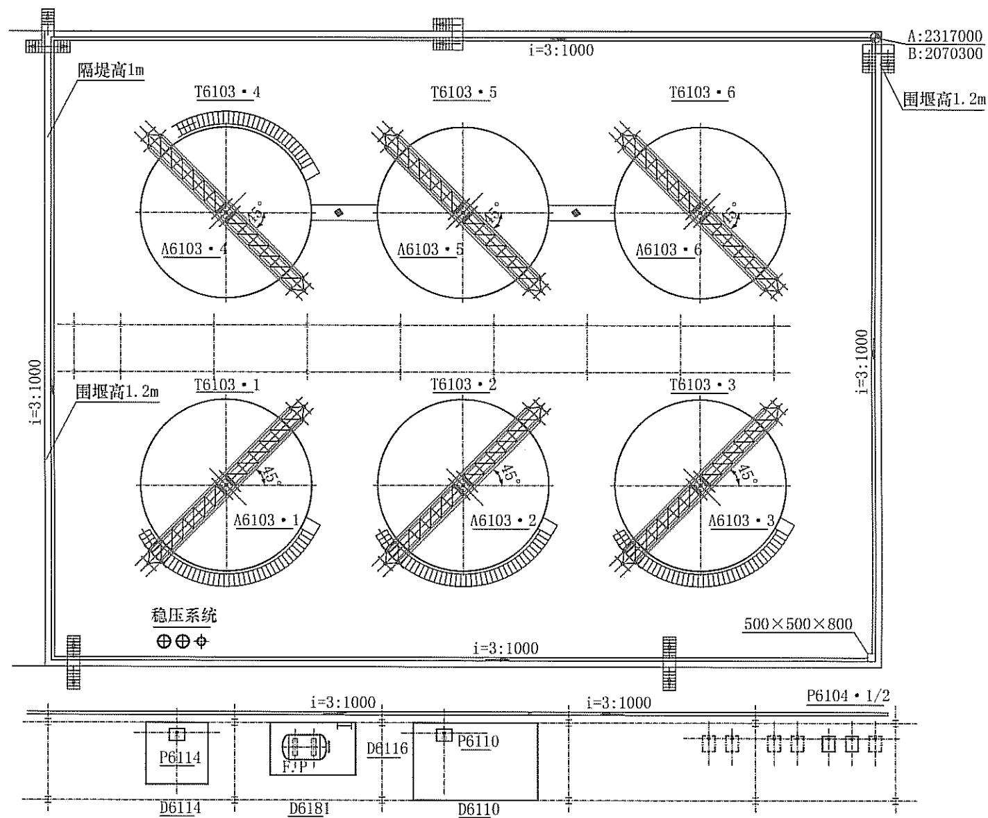
图 14.3.4 带有搅拌罐区的布置
