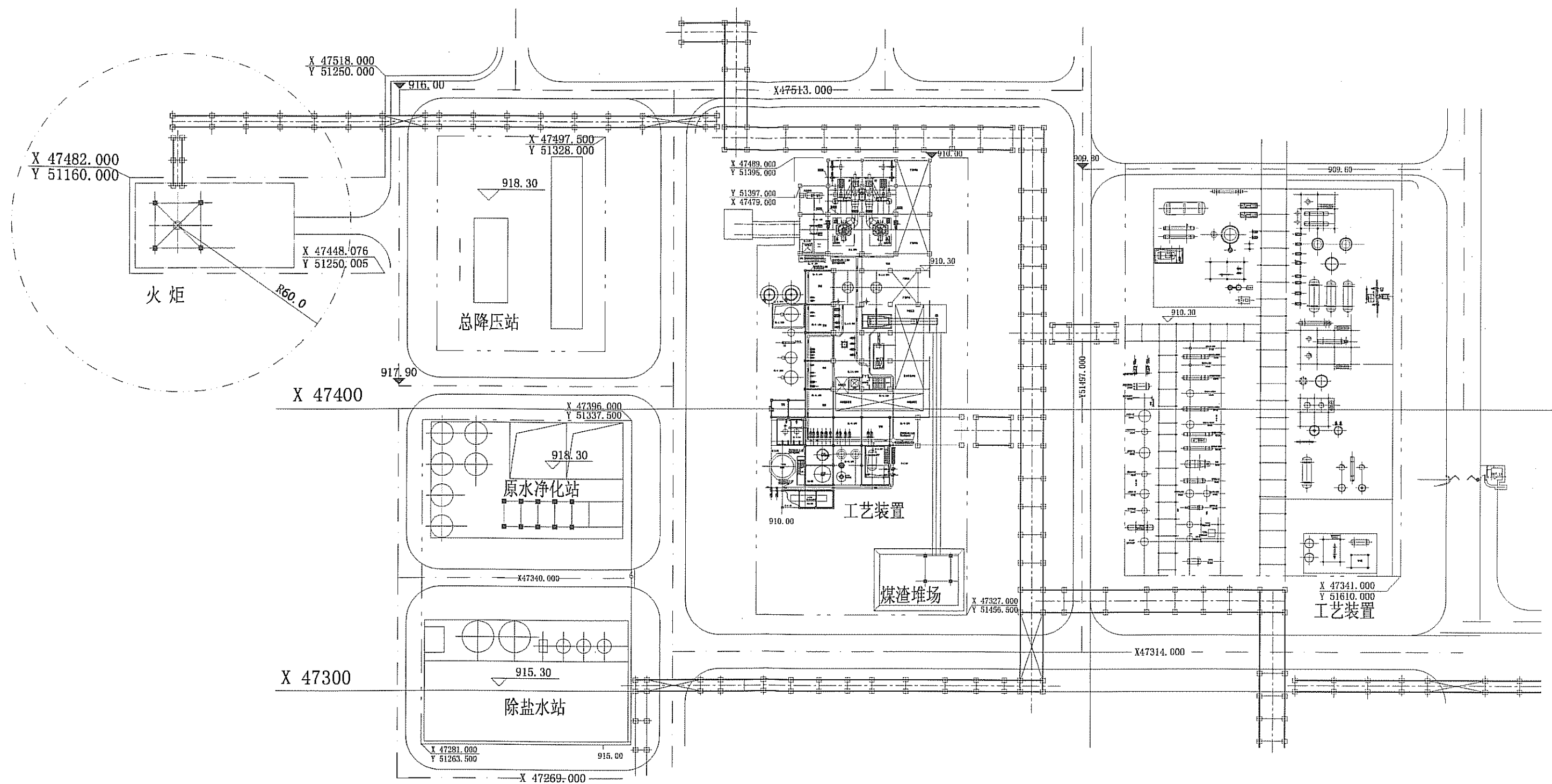
HG/T 20546.5—2009 图 12.3.5 外管架布置
